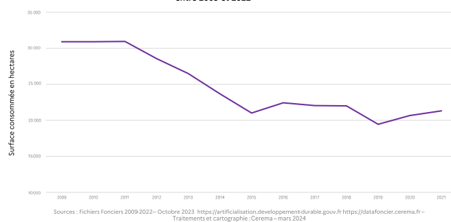
Evolution annuelle de la consommation d'espaces NAF en France entre 2009 et 2022
