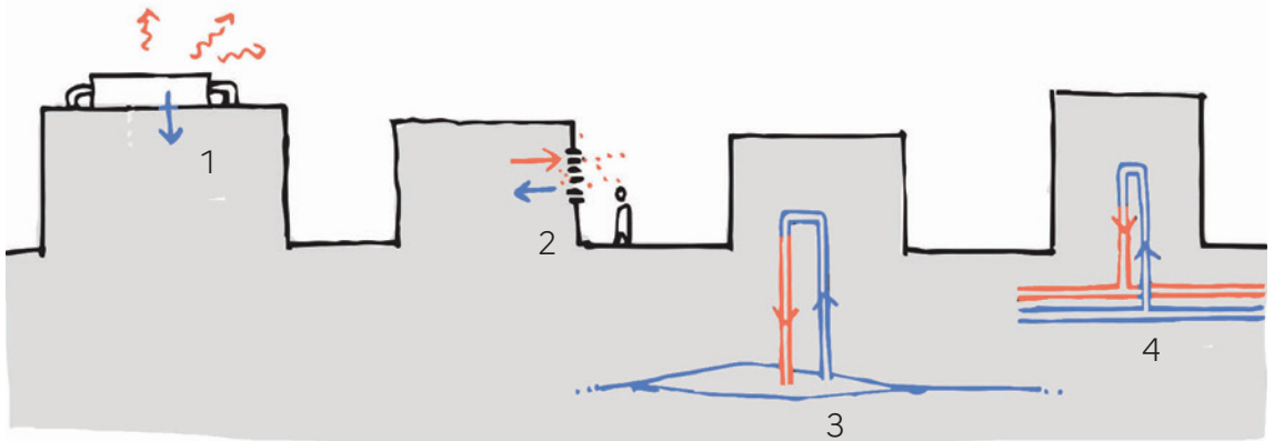
Les différents types de systèmes de rafraîchissement actifs
