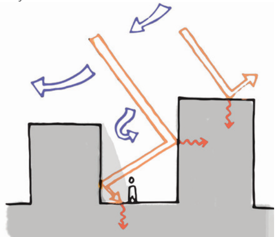
Piégeage du rayonnement solaire et écoulement de l'air perturbé par les obstacles construits qui empêche l'évacuation de chaleur la nuit, mais le jour l'ombrage améliore le confort.
