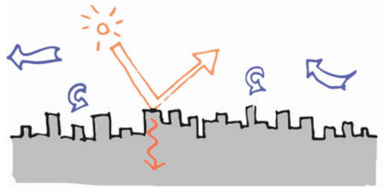
A grande échelle : la ville a un albédo effectif faible, la plupart des villes ont des albédos compris entre 0,15 et 0,2 et absorbent donc au moins 80% du rayonnement solaire.
